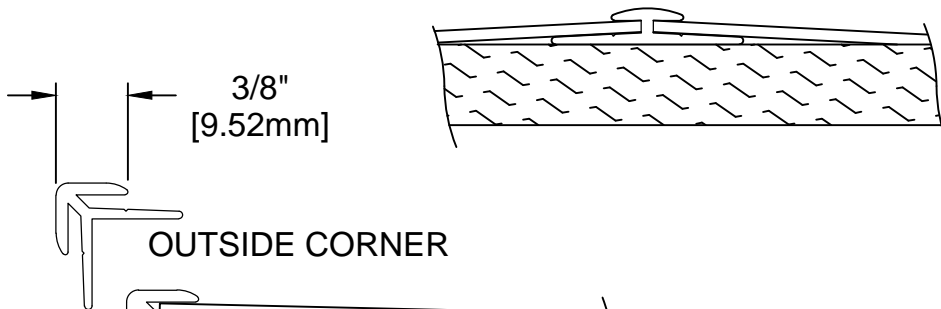
DIVIDER BAR
